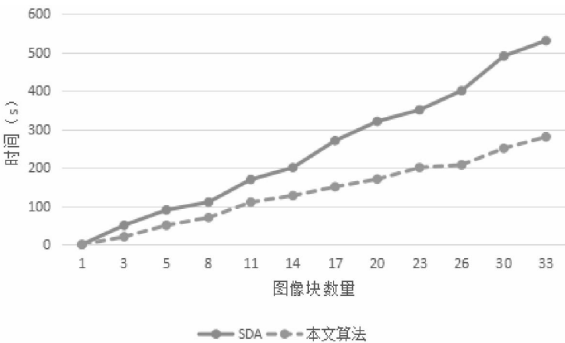
图3 时间复杂度对比图
