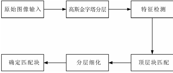
图 1 基于分层快匹配的图像配准算法流程图
